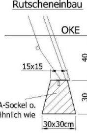
Fundamentschnitt Rutscheinbau
