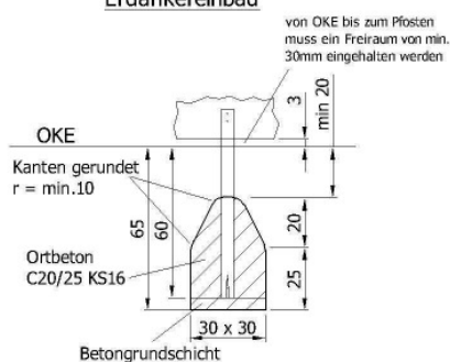
Fundamentschnitt Erdankereinbau
