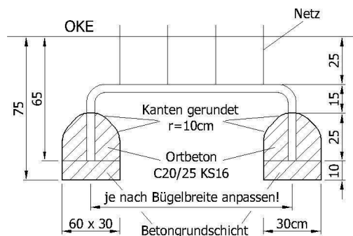
Fundamentalschnitt Rohrbügeleinbau
