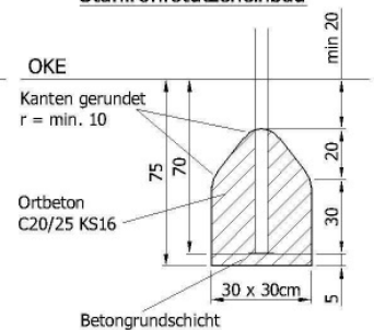
Fundamentschnitt Stahlrohrstützeinbau
