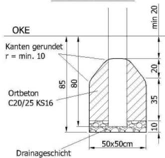
Fundamentschnitt Robiniererdeinbau
