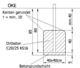
Fundamentschnitt Rutschstangeneinbau
