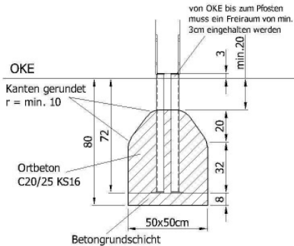
Fundamentschnitt Erdankereinbau
